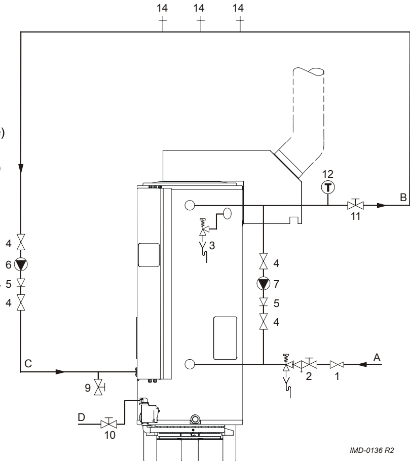
Schemat podłączeń
